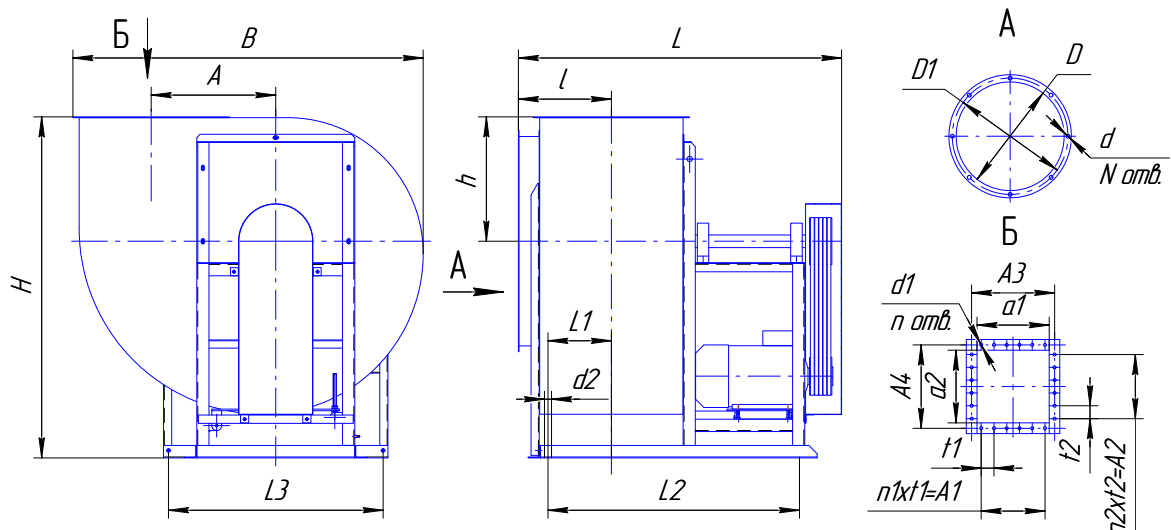
Исполнение 5-02
