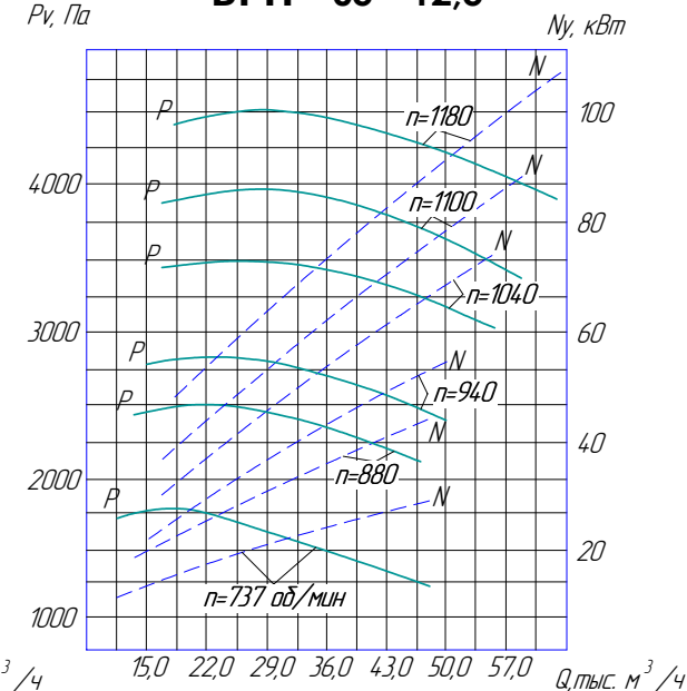
ВРП - 05 - 12,5
